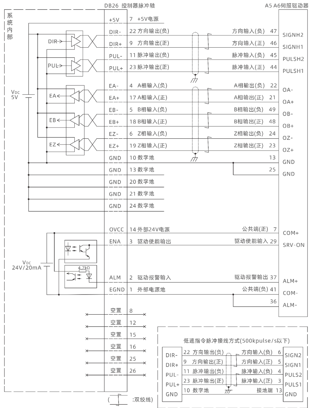
PUL/DIR 单端接线示意图：
