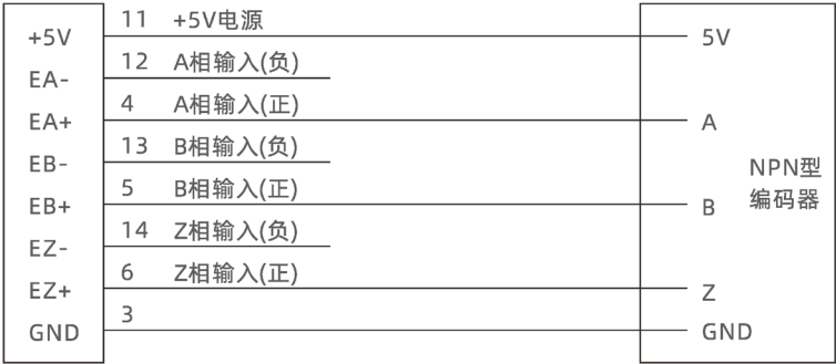
EA/EB/EZ 单端接线示意图:
