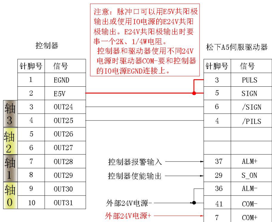
与松下 A5 单端接线参考
