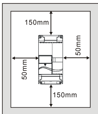
單機設置圖
