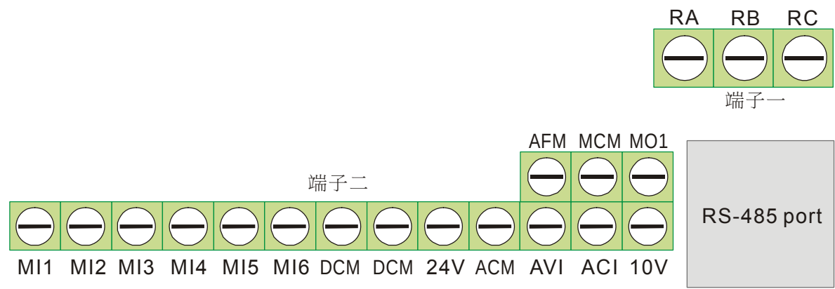
控制端子位置圖
