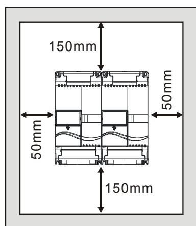
並排設置圖
