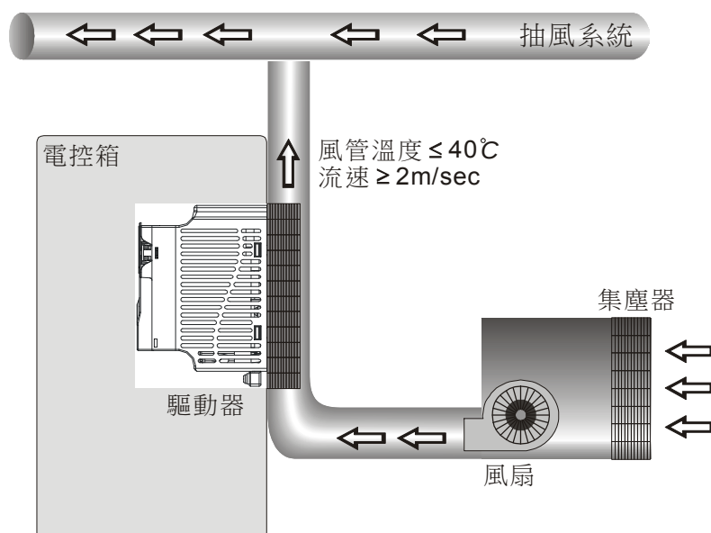
VFD-E-P 系列機種 散熱系統配置參考圖
