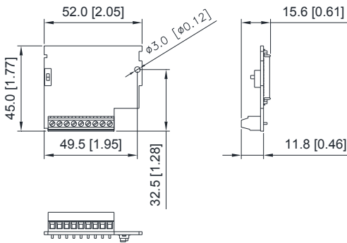
尺寸規格圖 Unit: mm [inch]
