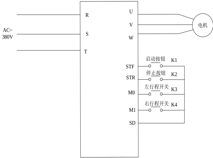
系统配线示意图
