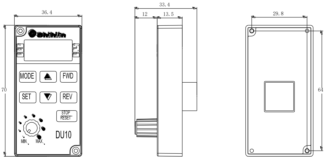
<外形尺寸图>
