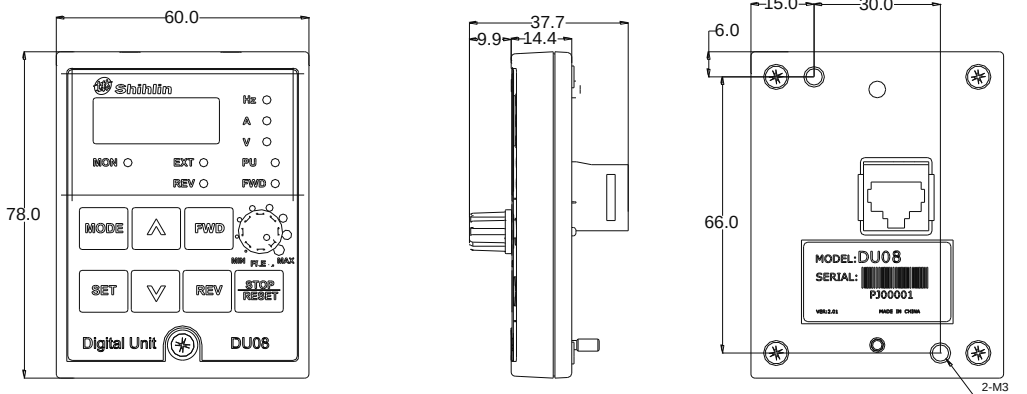
<盘面安装开孔尺寸图><法兰式安装开孔尺寸图(注)>
