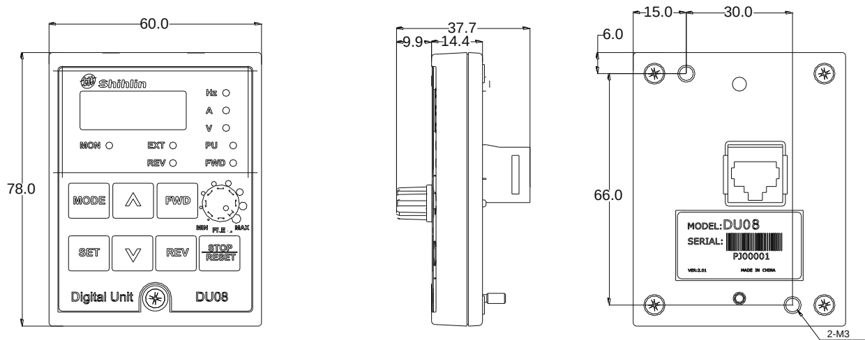
<外形尺寸图>
