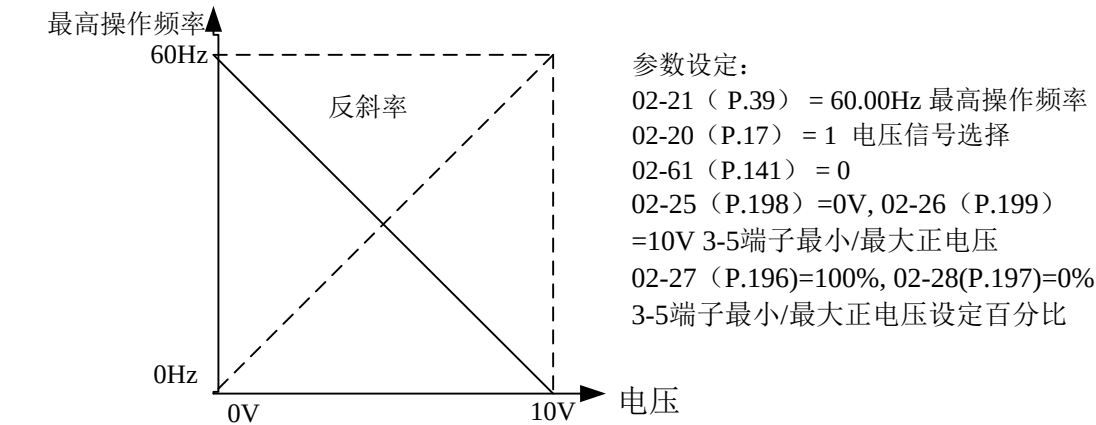
例 7：此范例是反斜率设定的应用。业界经常会使用一些感测器来做压力、温度、流量等的控制，而这些感测器有些是当压力大或流量高时，所输出的信号是 10V；而这个讯息就是要交流电机变频器减速或停止的命令，范例八的设定恰好满足此类的应用。
