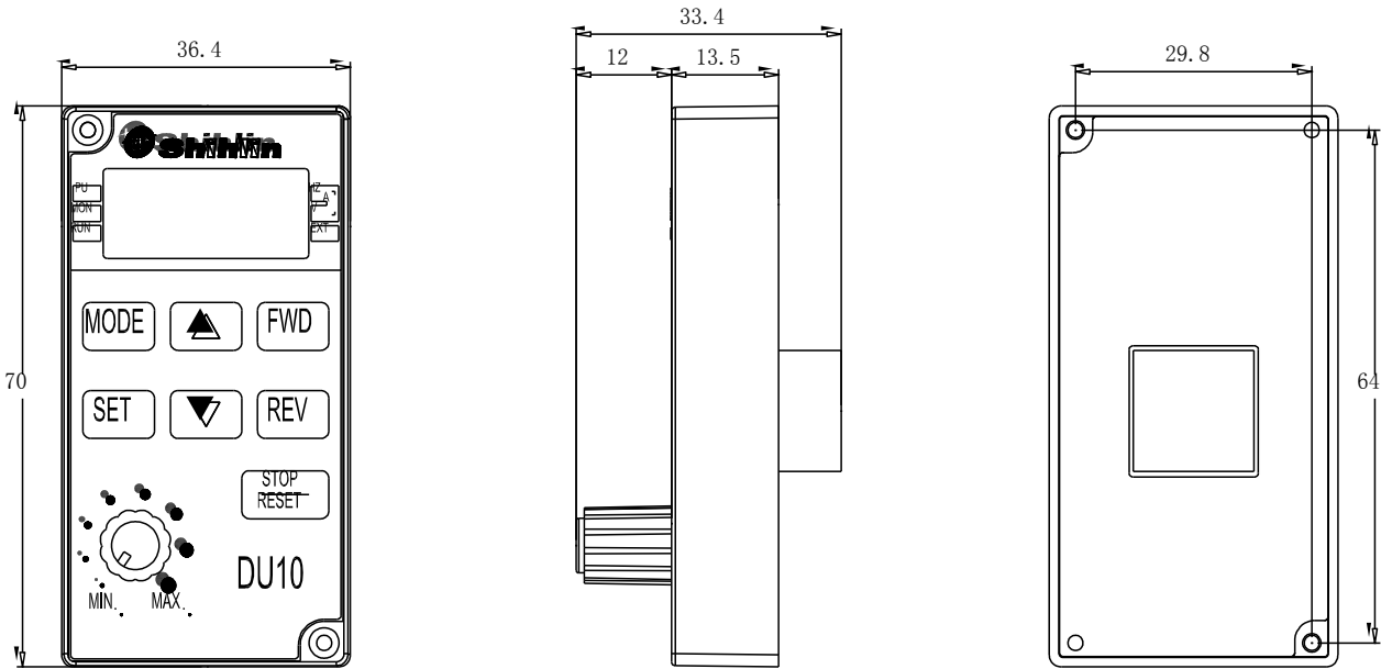
<外形尺寸图>
