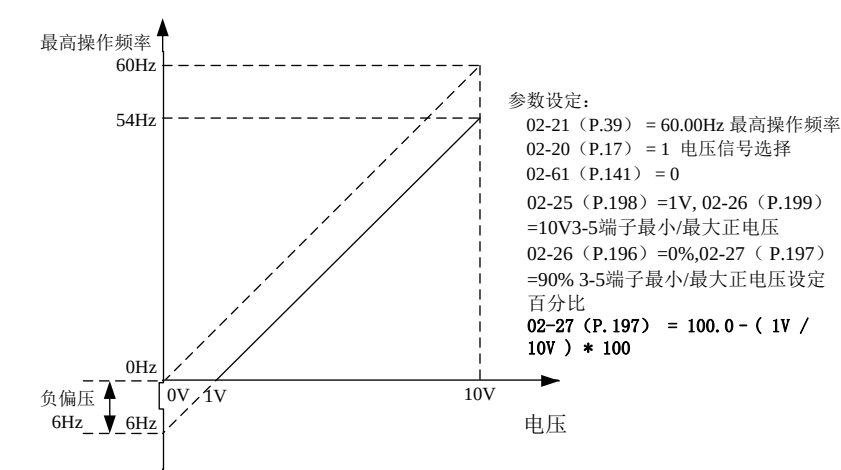
例 6：此范例是范例 5 的延伸。此类的应用极为广泛，使用者可以灵活应用。
